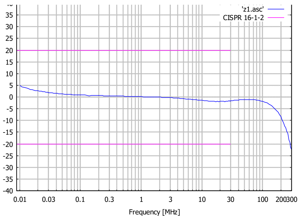
Bild 2: typ. Phasengang EuT Port, (Gleichtakt) Fig. 2: typ. phase EuT-port, (common mode)
