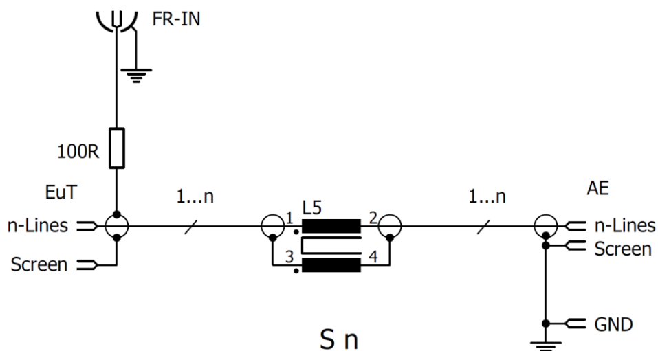
Bild 4: Prinzipschaltbild CDN ISN S1 BNC Fig. 4: principal circuitry CDN ISN S1 BNC
