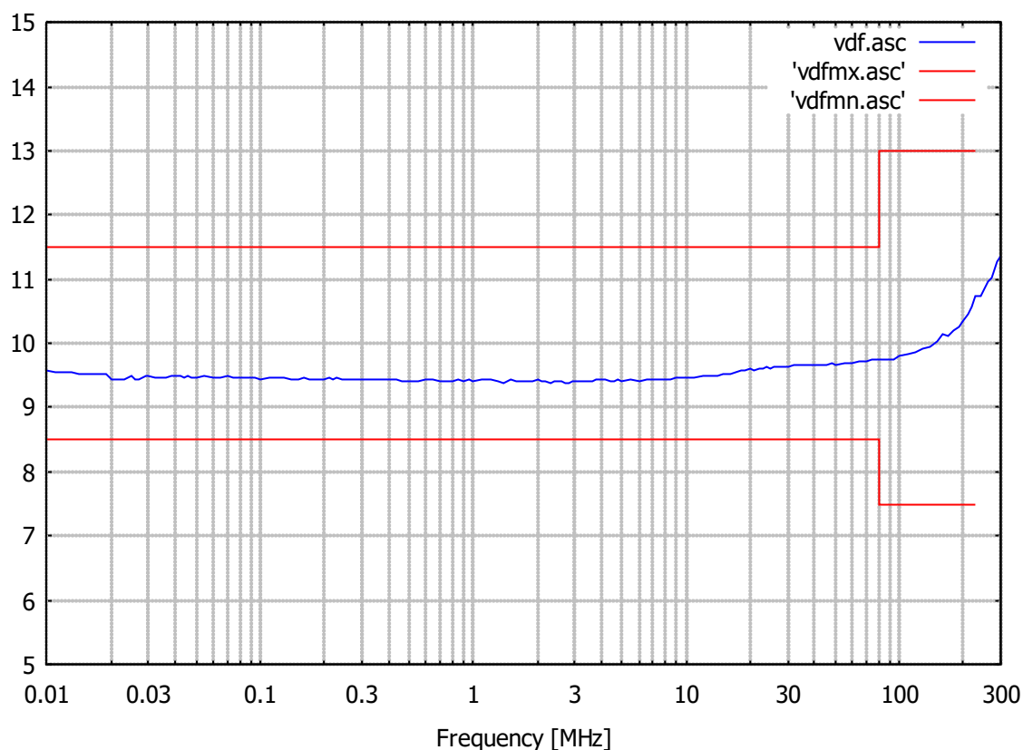
Bild 3: typ. Spannungsteilungsfaktor HF-Port zu EuT-Port Fig. 3: typ. voltage division factor RF-port to EuT-port
